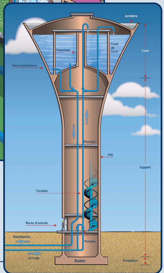
Coupe d'un réservoir
