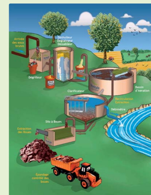
Station d'épuration par boues activées
